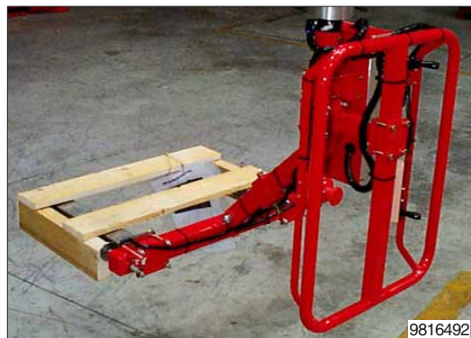
Display-pallets ook met producten te verplaatsen. De contactsensor zorgt voor een veilige opname.
