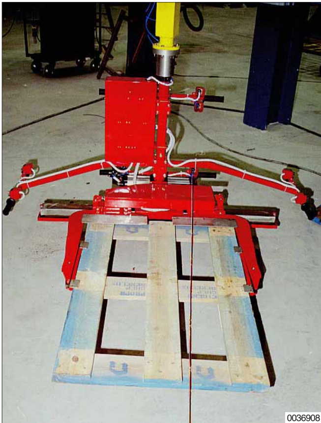
Het klemmend opnemen en pneumatisch draaien van afdek-pallets.
