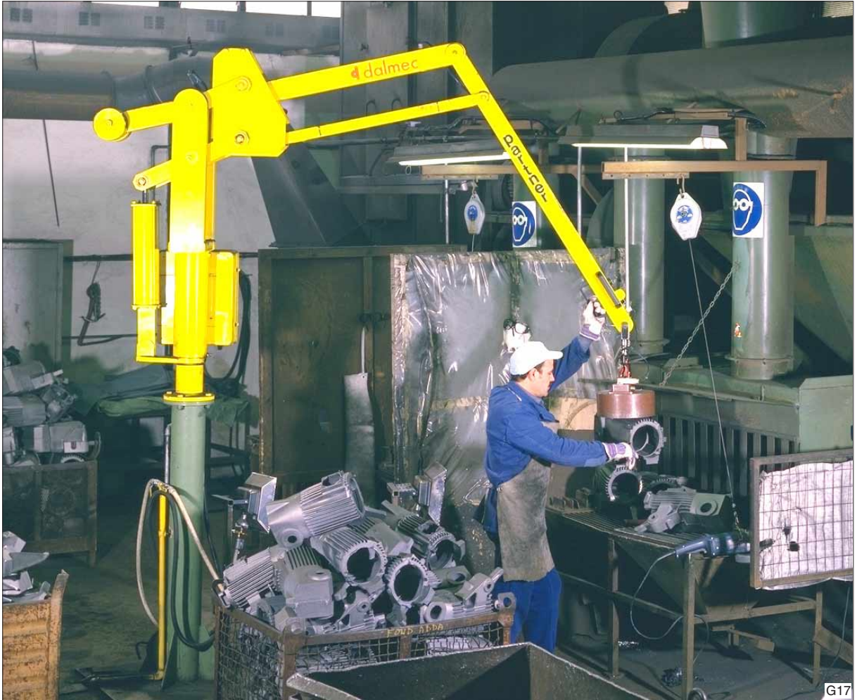
Een permanent magneet voor het opnemen van stalen behuizingen van een elektromotor. In combinatie met de Dalmeccan Partner balancer, type PSC, krijgt onaangenaam werk meer inhoud.
