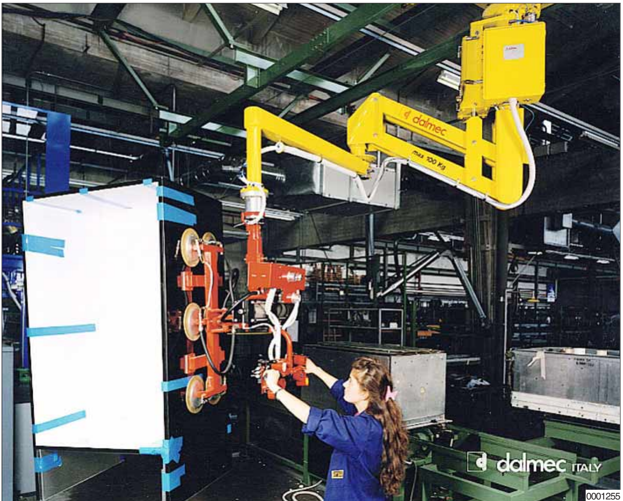
Dalmec Partner balancer, hangend verrijdbaar, voorzien van een lastopnemer met zes zuigschalen voor het handlen van de ombouw van een koelkast. Schijnbaar gewichtloos, dus moeiteloos en licht.
